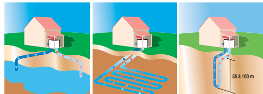
Captage sur nappe Captage horizontal Captage vertical
